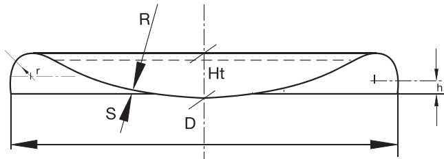
Diffuseurböden
