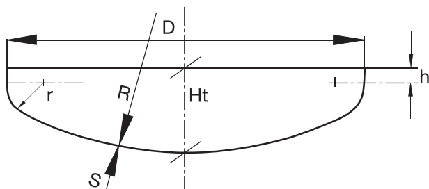
Fonds bombés a grand rayon de carre (grc) (p. 18-19)
